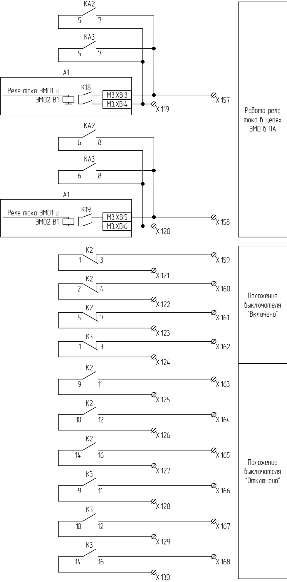
Выходные цепи
